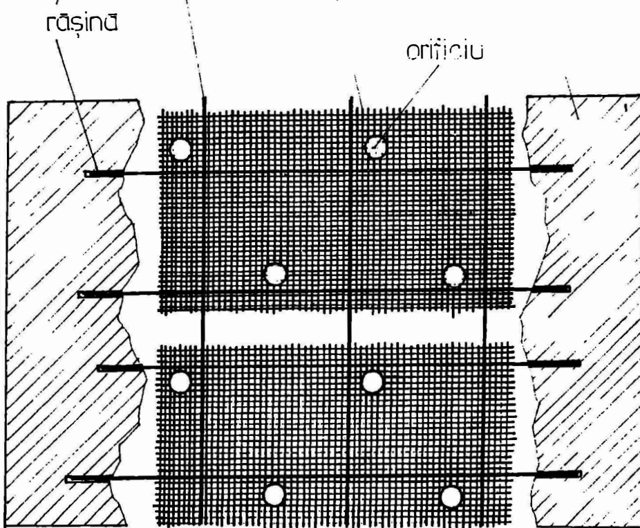
Secțiune longitudinală prin plombă
