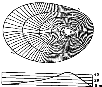
Fig. 6 și 7. O movilă, reprezentată prin hașure și curbe de nivel. După SEYDLITZ.
