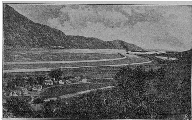
Fig. 24. Canalul Dunării la Porțile de fer.
