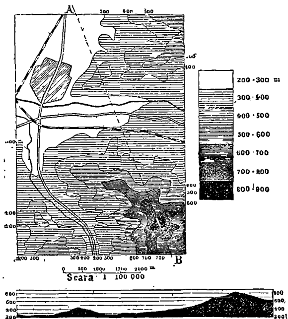
Fig. 8. Sus. O hartă lucrată în curbe de nivel. Jos. O secțiune verticală dealungul liniei A-B construită prin ajutorul curbelor de nivel.
