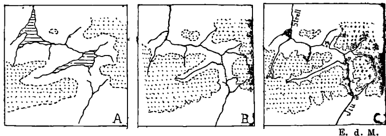
Fig. 38. Schemă de schimbările Jiului, din epoca neogenă (terțiară) A și actuală C. Ce-î punctat e peste 1000 m. H=Hațeg, M=Curmătura Merișor, P=Petroșani, L=Lainici, B=Bumbești.
