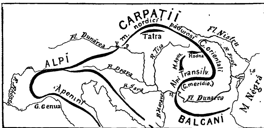
Fig. 9. Schiță orografică simplificată a Europei centrale.
