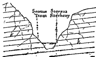
Fig. 37. Secțiune în Clisura Cazan.
