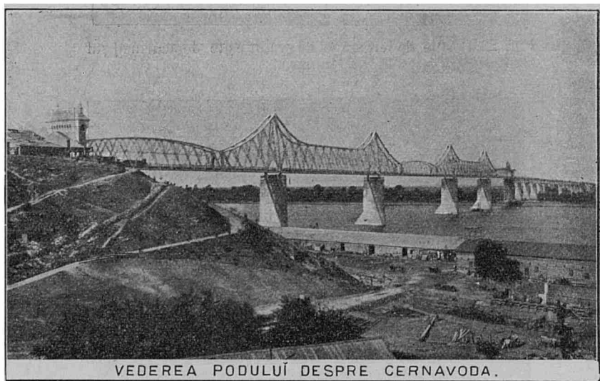
Fig. 26. Podul «Carol I.» peste Dunăre. Calea ferată duce de la București prin Fetești la Constanța.
