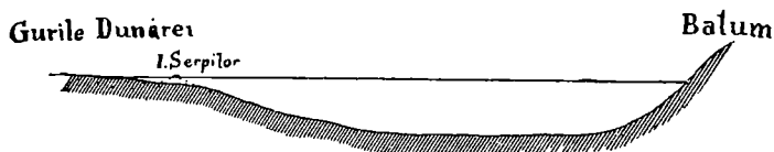
Fig. 23. Secțiune prin Marea Neagră, de la V la E.
