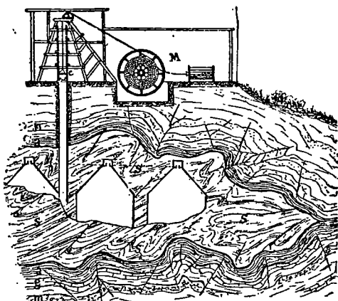
Fig. 47. Vederea unui masiv de sare în exploatațiune. n , nisip; a , argile; s , sare; g , gips; m , marne.
