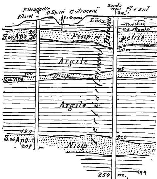
Fig. 25. Secțiune prin subsolul Bucurescilor.
