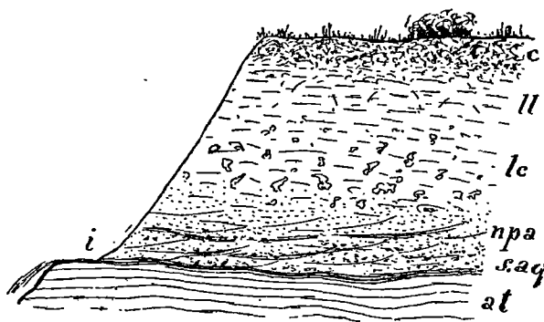
Fig. 43 Tăetură prin solul arabil de pe câmpia Munteniei c. humus (cernoizem) ll. löss levigat (spălat) lc löss cu concrețiuni; npa. nisip, pietriș, intercalațiuni de argile, saq. strat aquifer; at. argile terțiare. i. izvor.
